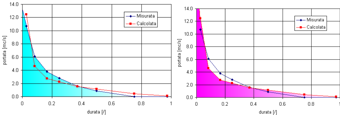
Illustrazione 19: Rappresentazione della curva di durata calcolata (a sinistra) e misurata (a destra) e della rispettiva area sottesa. Le curve sono riferite al periodo estivo
